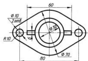
Деталь «крышка»
