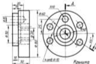
Рисунок 7 – Деталь «крышка»
