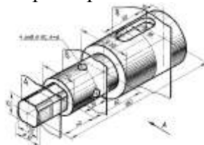
Рисунок 8 – Деталь «вал»
