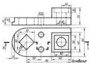
Рисунок 6 – Деталь «основание»
