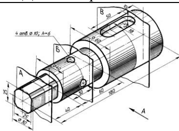
Деталь «вал»
